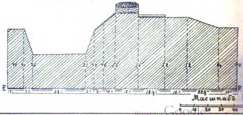
№ 3. Профиль по Линіи Е. Ф.
